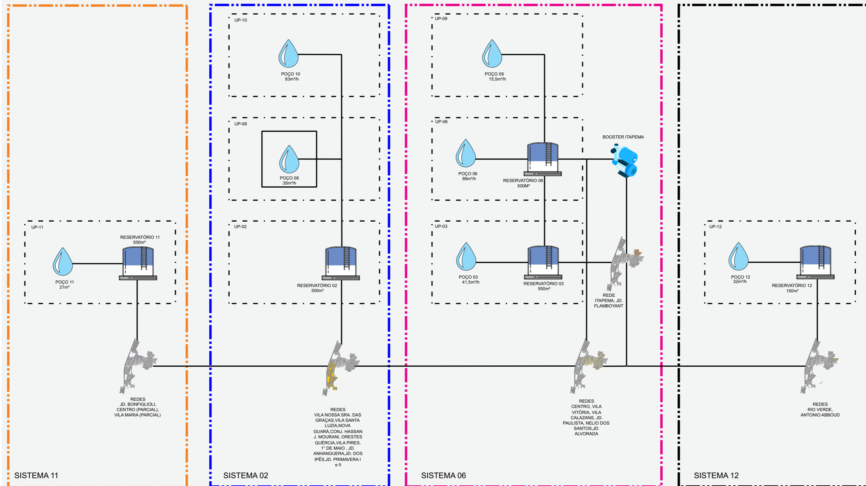
SAA - DIAGNÓSTICO - FLUXOGRAMA DE ÁGUA - GUARÁ / SEDE
